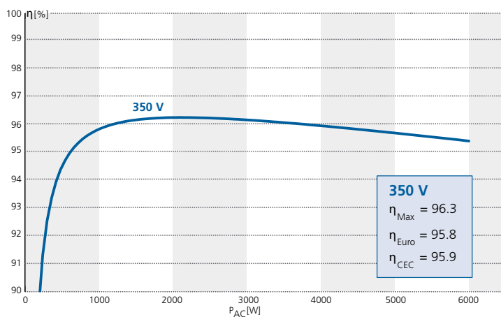
Wirkungsgradkennlinie Powador 6600
