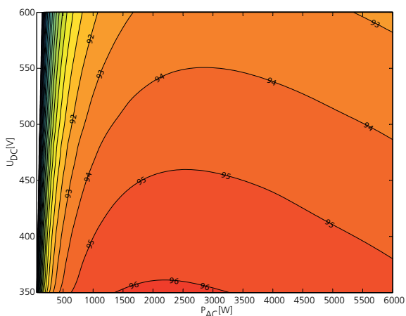
3D-Wirkungsgraddiagramm Powador 6600
